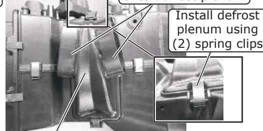
Defrost Plenum 625321
